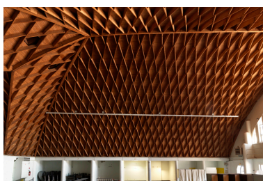
Vue intérieure vers l'ouest. La charpente et les loges des bas-côtés. Phot. Thierry Lefébure IVR32_20208000149NUC2AQ
