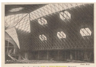
La halle en construction. Extrait de CRESTIN, F. "Les charpentes en lamelles de bois...". Le Génie civil : revue générale des industries françaises et étrangères , 1933. Phot. Archives départementales de la Somme IVR32_20168006552NUCA
