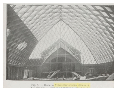
La halle en construction. Extrait de CRESTIN, F. "Les charpentes en lamelles de bois...". Le Génie civil : revue générale des industries françaises et étrangères , 1933. Phot. Archives départementales de la Somme IVR32_20168006551NUCA
