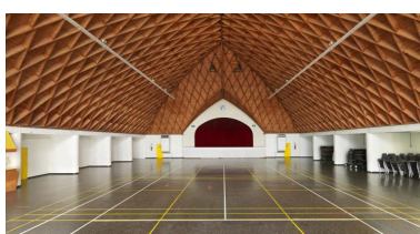
Vue intérieure vers le sud. Phot. Thierry Lefébure IVR32_20218000005NUCAQ
