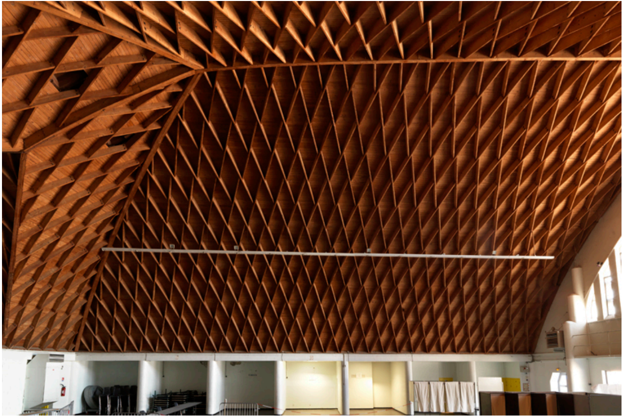
Vue intérieure vers l'ouest. La charpente et les loges des bas-côtés.
