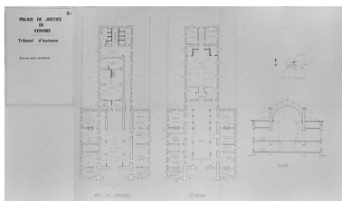
Plans par niveau, vers 1970. Phot. Pierre-Yves Brest (reproduction) IVR22_19970202505ZB
