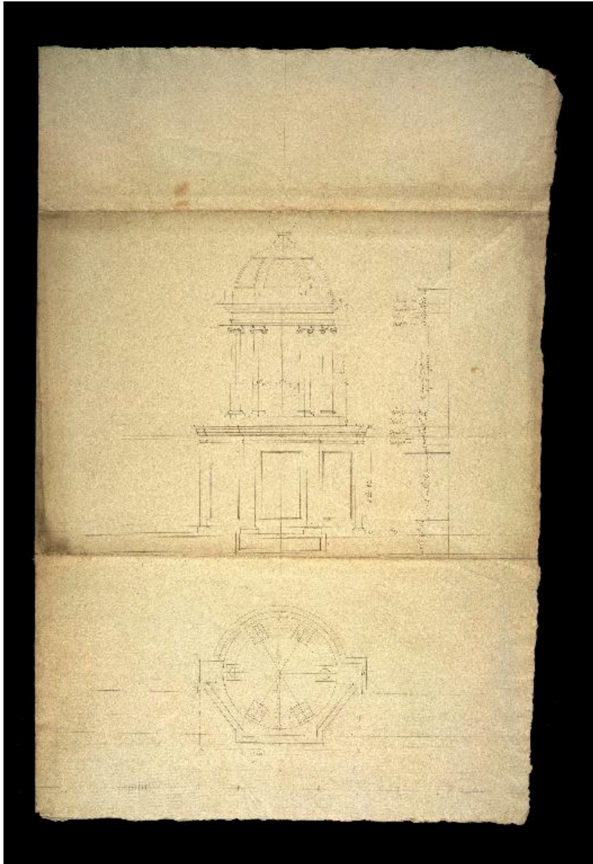
Élévation et coupe du tabernacle à dais du maître-autel, dessinées par l'architecte Carrier vers 1807 (A Évêché Soissons : P Soissons-Cathédrale, 3 D).
