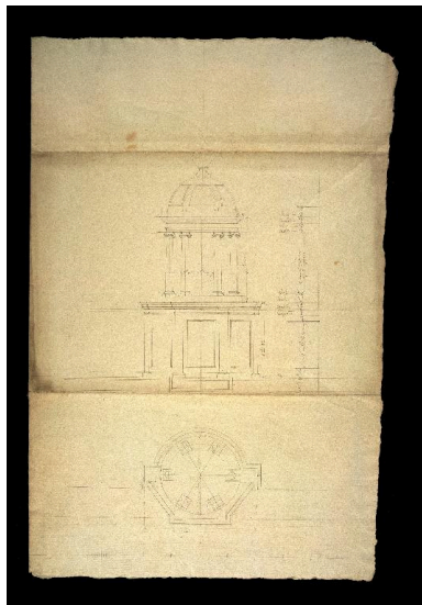
Élévation et coupe du tabernacle à dais du maître-autel, dessinées par l'architecte Carrier vers 1807 (A Évêché Soissons : P Soissons-Cathédrale, 3 D). Phot. Leullier Irwin IVR22_20020200539XAB
