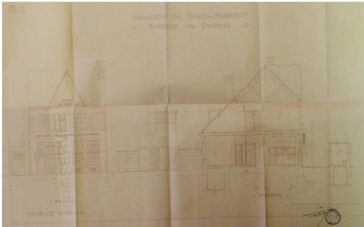
Bureau de postes, élévation et coupe, 1934 (AD Somme ; 99 O 3366).
