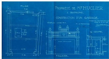
Propriété de M. Huclier à Bapaume - construction d'un garage. Signé et daté par Paul Auger, architecte, et E. Huclier, propriétaire, le 10 Mai 1926. (AD Pas-de-Calais, 10R9/40, dossier n°589). Phot. Thibaut Pierre (reproduction) IVR32_20216200011NUCA
