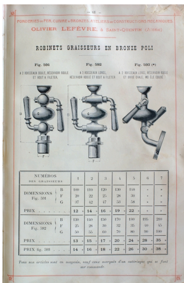
Robinet graisseurs en bronze poli, 1902 (AC Saint-Quentin). Phot. Pillet Frédéric IVR22_20050205797NUCAB
