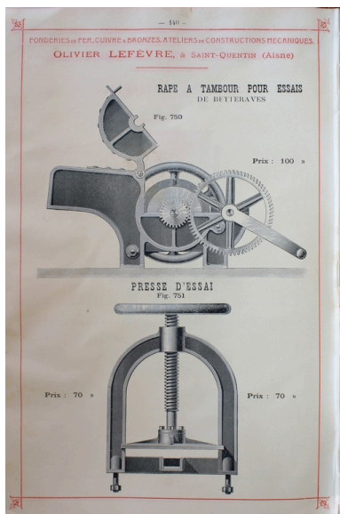
Râpe à tambour pour essais de betteraves, et presse d'essai, 1902 (AC Saint-Quentin). Phot. Pillet Frédéric IVR22_20050205799NUCAB
