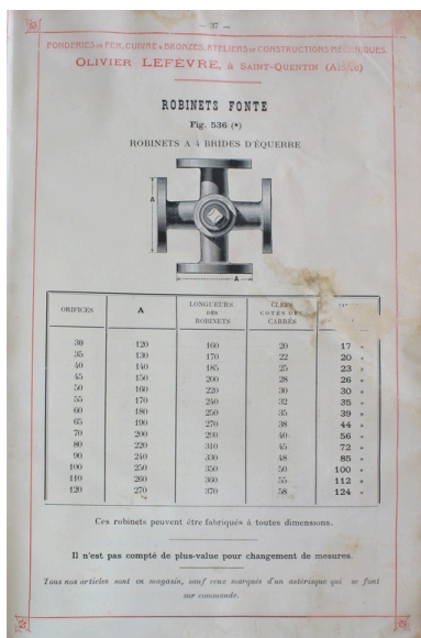
Robinet fonte à quatre brides d'équerre, 1902 (AC Saint-Quentin). Phot. Pillet Frédéric IVR22_20050205796NUCAB
