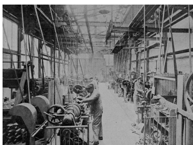
Vue d'ensemble de l'atelier de mécanique reconstitué, 1920-1922 (Le Monde Illustré). Phot. Pillet Frédéric IVR22_20050205809NUCAB
