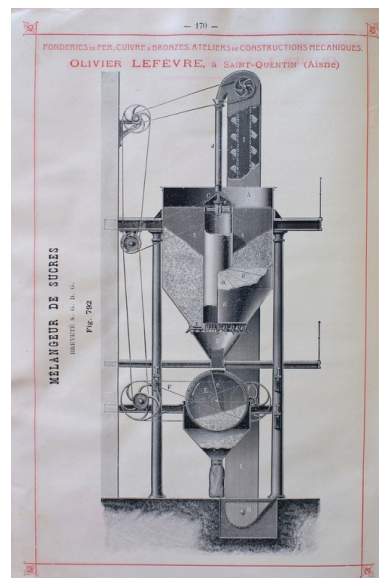
Mélangeur de sucres, 1902 (AC Saint-Quentin). Phot. Pillet Frédéric IVR22_20050205801NUCAB
