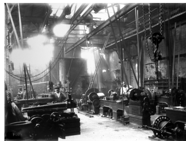
Atelier dit de mécanique (atelier d'usinage) vers 1919-1920 (AD Aisne). Phot. Pillet Frédéric IVR22_20050205813NUCAB
