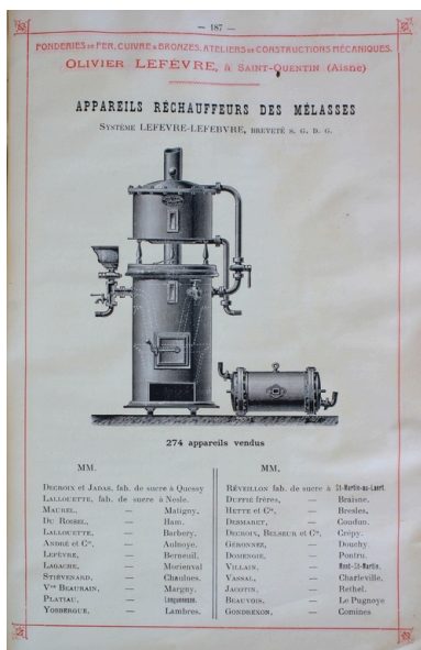
Appareils réchauffeurs des mélasses, 1902 (AC Saint-Quentin). Phot. Pilet Frédéric IVR22_20050205802NUCAB
