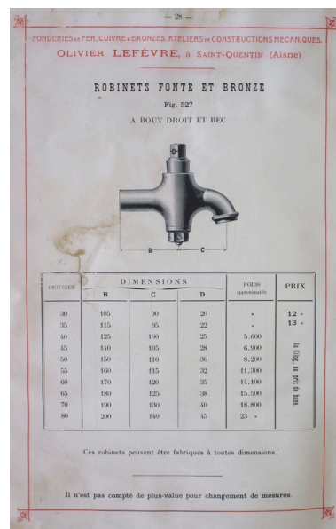
Robinet fonte et bronze à bout droit et bec, 1902 (AC Saint-Quentin). Phot. Pilet Frédéric IVR22_20050205795NUCAB
