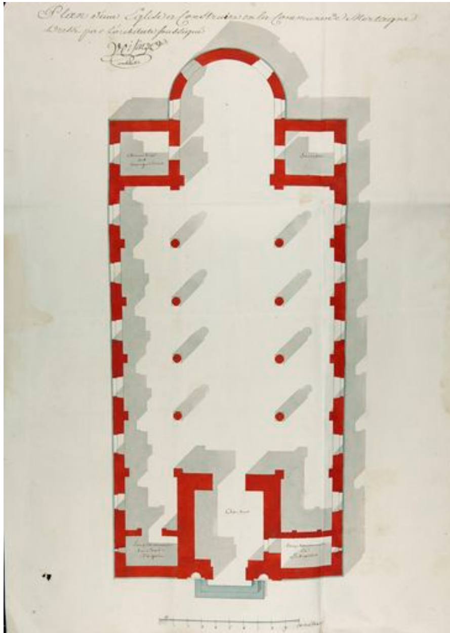
Plan de l'église projetée, Voisin architecte, 1820 (AD Nord 20421-72).
