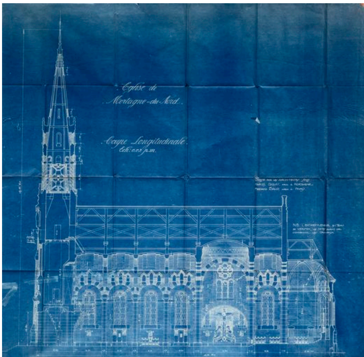
Coupe de l'église, Fernand Baud et Marcel Coquet architectes, 1924 (AD Nord, 20421/200).
