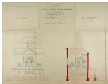
Elévation postérieure, Paul Destombes architecte, 1888 (AD Nord 20421-83). Phot. Hubert Bouvet IVR31_20105900569NUCA
