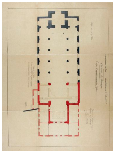
Plan du projet d'agrandissement, Paul Destombes architecte, 1888 (AD Nord 20421-83). Phot. Hubert Bouvet IVR31_20105900568NUCA
