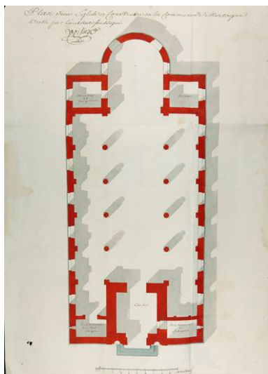
Plan de l'église projetée, Voisin architecte, 1820 (AD Nord 20421-72). Phot. Hubert Bouvet IVR31_20105900556NUCA
