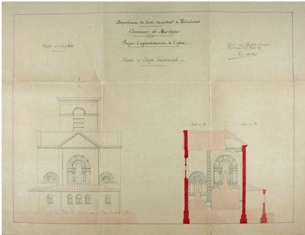
Elévation postérieure, Paul Destombes architecte, 1888 (AD Nord 2O421-83).
