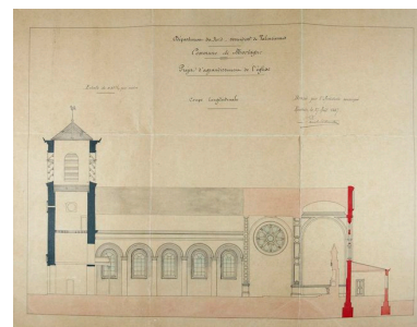
Coupe transversale, Paul Destombes architecte, 1888 (AD Nord 20421-83). Phot. Hubert Bouvet IVR31_20105900567NUCA
