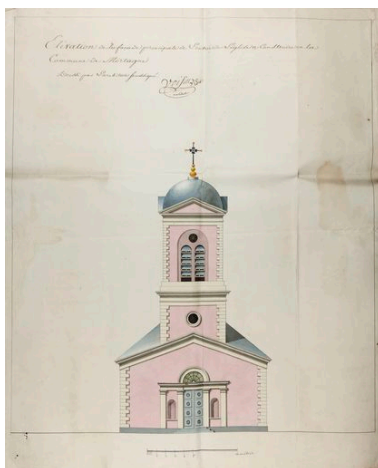
Elévation antérieure de l'église projetée, Voisin architecte, 1820 (AD Nord, 20421-72). Phot. Hubert Bouvet IVR31_20105900557NUCA
