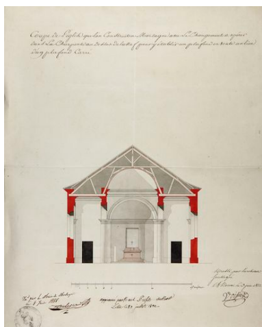
Coupe de l'église projetée, Voisin architecte (AD Nord 20421-72). Phot. Hubert Bouvet IVR31_20105900561NUCA
