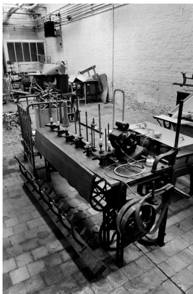
Bobinoirs, constructeur inconnu. Phot. Benoît Dufournier IVR22_19878000443Z
