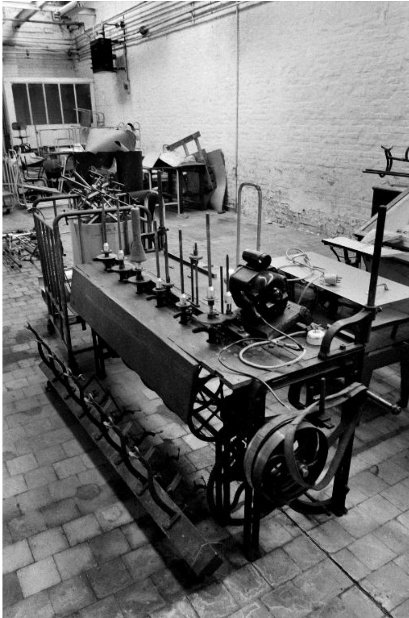
Bobinoirs, constructeur inconnu.
