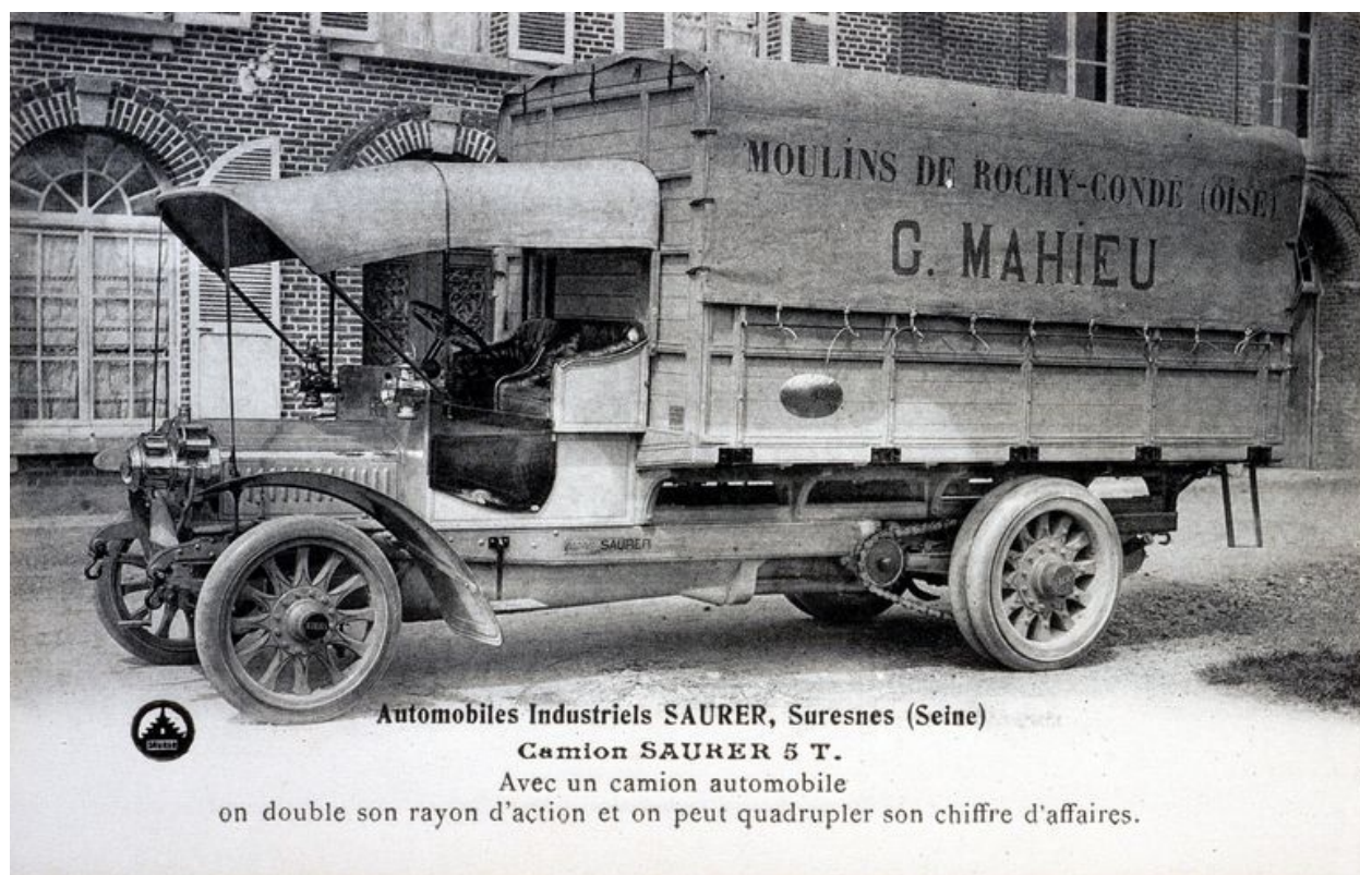
Le camion Saurer 5 T de la minoterie Mahieu, vers 1914. (Carte postale, coll. part.).
