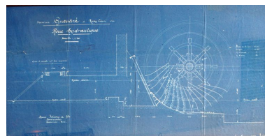
Coupe de la roue hydraulique. Phot. Fournier Bertrand (reproduction) IVR22_20046003077NUCAB
