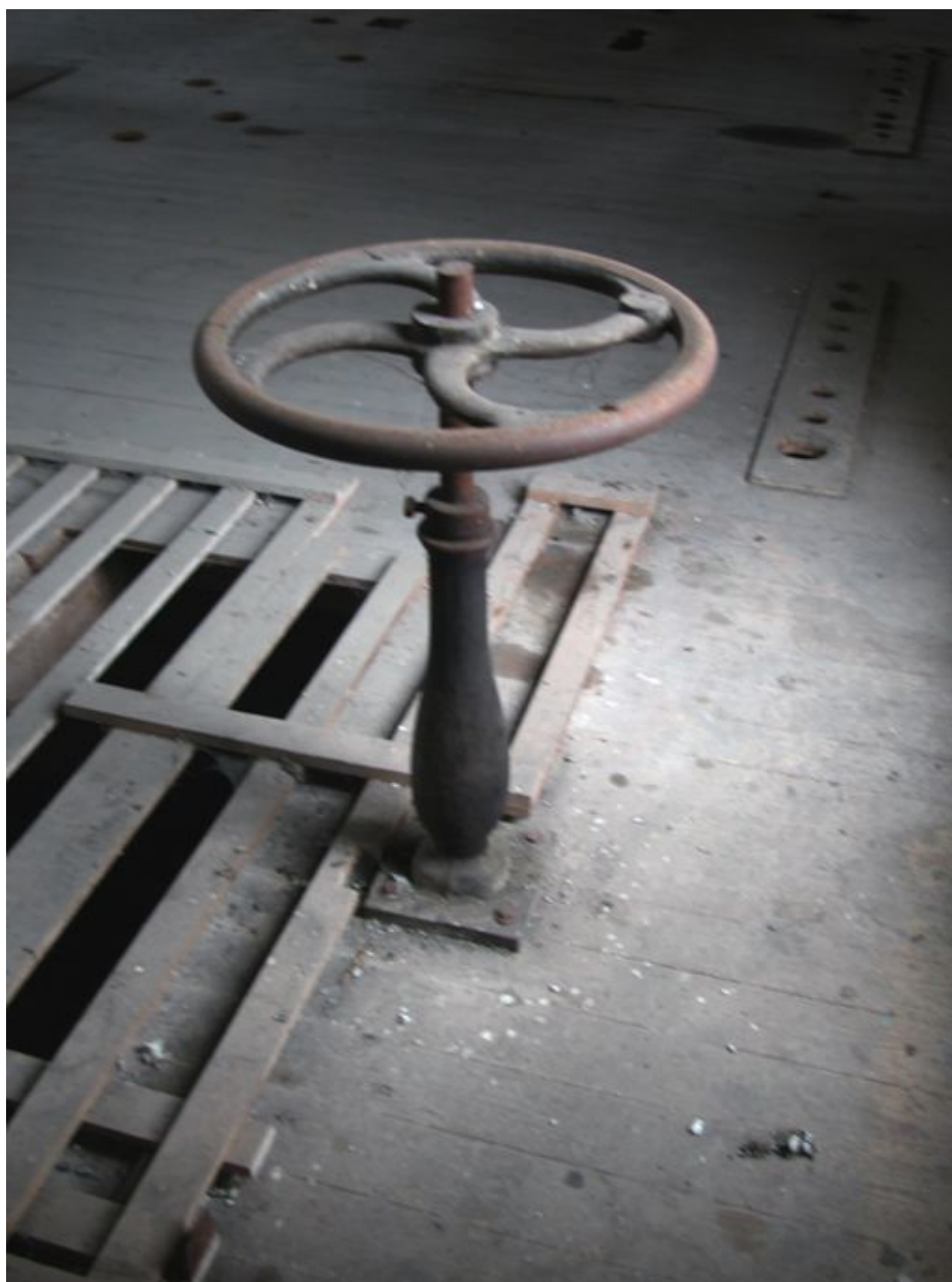
Intérieur du premier étage, détail du volant de commande d'ouverture de la vanne moulinaire.
