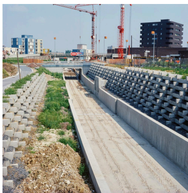
La construction de la ligne de métro au Triolo, en tranchée
