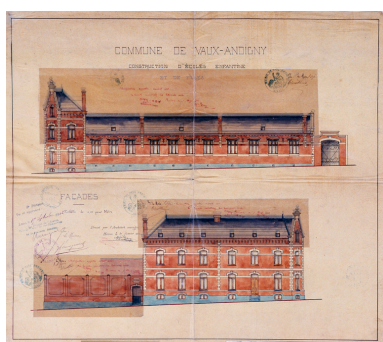
Commune de Vaux-Andigny. Construction d'une école enfantine et de filles. Elévations sur rue, Désiré Leroy architecte, 1902 (AD Aisne ; AC, Vaux-Andigny : 4 M 3). Phot. Thierry Lefébure IVR22_19920200121XAB
