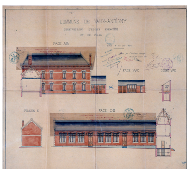
Commune de Vaux-Andigny. Construction d'une école enfantine et de filles. Elévations sur la cour, Désiré Leroy architecte, 1902 (AD Aisne ; AC, Vaux-Andigny : 4 M 3). Phot. Thierry Lefébure IVR22_19920200120XAB
