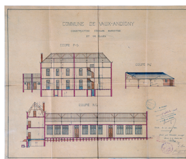
Commune de Vaux-Andigny. Construction d'une école enfantine et de filles. Coupes, Désiré Leroy architecte, 1902 (AD Aisne ; Vaux-Andigny : 4 M 3). Phot. Thierry Lefébure IVR22_19920200122XAB
