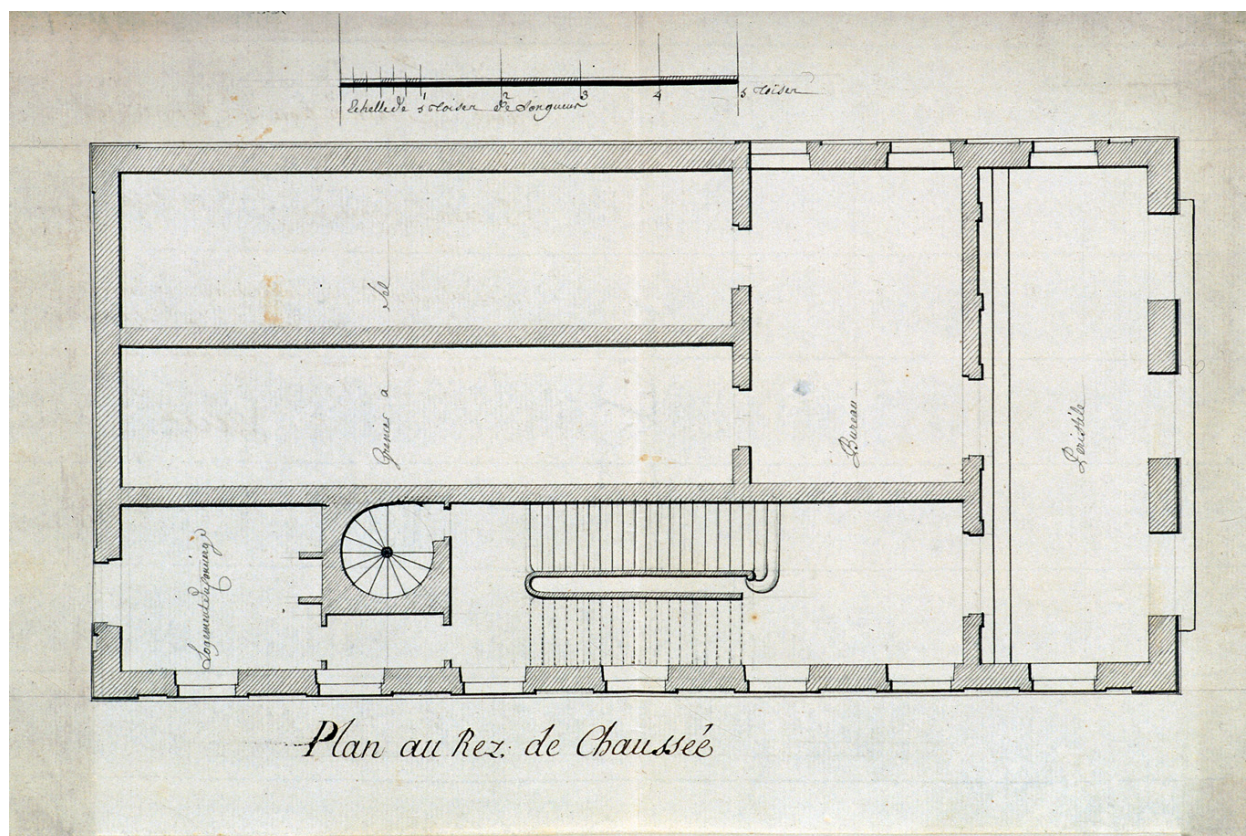
Hôtel de ville de Roye : plan du rez-de-chaussée, 1770 (AD Somme ; 1C_CP_1062/29).
