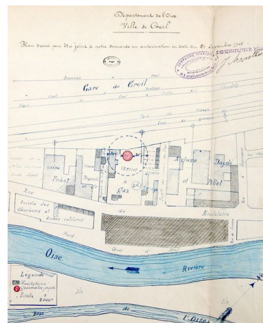
Plan de l'usine à gaz et de ses gazomètres, 1907 (AD Oise ; 5Mp2456/1). Phot. Clarisse Lorieux IVR22_20076005065NUCAB
