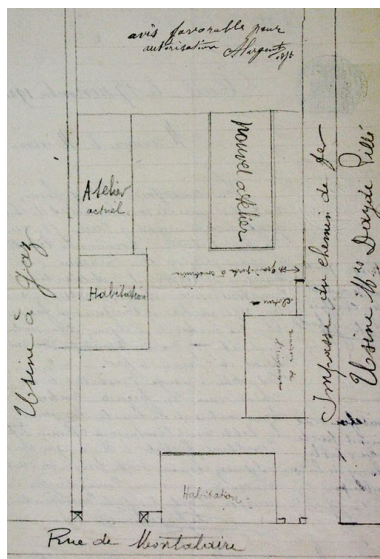
Plan de situation de la scierie Lepage et du nouvel atelier à construire, 1903 (AC Creil ; 101 65). Phot. Clarisse Lorieux IVR22_20076005452NUCAB
