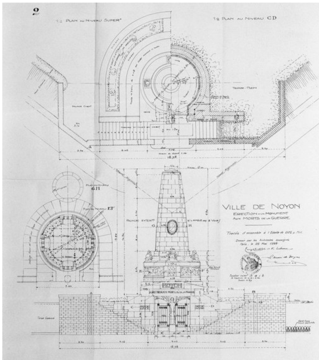
Plan du 2e niveau et élévation antérieure, par E. Chifflet et R. Lefevre, 1924 (AD Oise ; série O).
