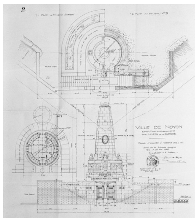
Plan du 2e niveau et élévation antérieure, par E. Chifflet et R. Lefevre, 1924 (AD Oise ; série O). Phot. Jean-Michel Périn IVR22_19846000364XB
