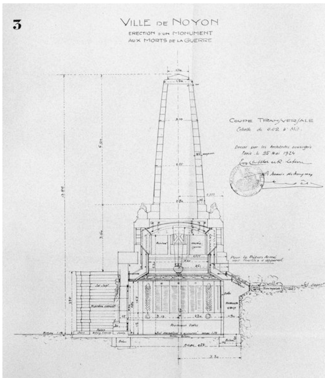
Coupe transversale, par E. Chiffot et R. Lefevre, 1924 (AD Oise ; série O).
