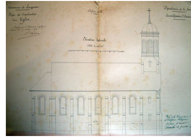
Longueau. Projet de construction d'une église. Élévation latérale, Henry Antoine architecte, 1849 (AD Somme ; 99 O 2405) Repro. Isabelle Barbedor IVR22_20058010500NUCA
