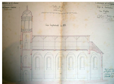
Longueau. Projet de construction d'une église. Coupe longitudinale, Henry Antoine architecte, 1849 (AD Somme ; 99 O 2405) Repro. Isabelle Barbedor IVR22_20058010502NUCA
