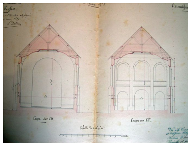
Longueau. Projet de construction d'une église. Coupes transversales, Henry Antoine architecte, 1849 (AD Somme ; 99 O 2405) Repro. Isabelle Barbedor IVR22_20058010501NUCA
