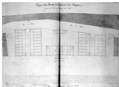
Douane, entrepôt public, plan du rez-de-chaussée, éch. 0,01 p.m. B.M. Boulogne-sur-Mer, ms 535 P. pl. 7. Repro. Philippe Dapvril IVR31_19946200056X
