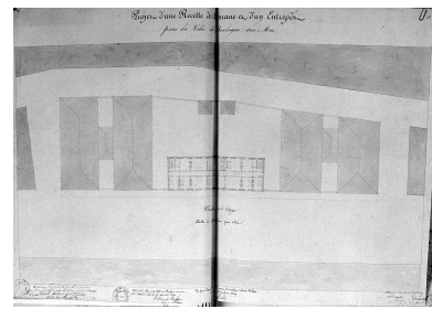
Douane, entrepôt public, plan du 2e étage, éch. 0,01 p.m. B.M. Boulogne-sur-Mer, ms 535 P. pl. 11. Repro. Philippe Dapvril IVR31_19946200058X
