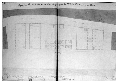
Douane, entrepôt public, plan du 1er étage, éch. 0,01 p.m. B.M. Boulogne-sur-Mer, ms 535 P. pl. 9. Repro. Philippe Dapvril IVR31_19946200057X
