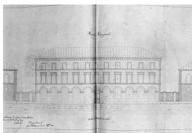
Douane, entrepôt public, façade sur quai, plan éch. 0,01 p.m. B.M. Boulogne-sur-Mer, ms 535 P. pl. 15 part. Repro. Philippe Dapvril IVR31_19946200067X
