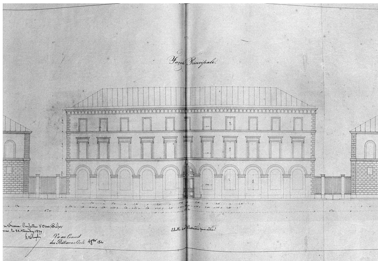
Douane, entrepôt public, façade sur quai, plan éch. 0,01 p.m. B.M. Boulogne-sur-Mer, ms 535 P. pl. 15 part.
