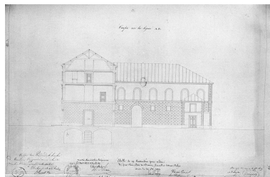
Douane, entrepôt public, coupe façade A-B, éch. 0,01 p.m. B.M. Boulogne-sur-Mer, ms 535 P. pl. 13. Repro. Philippe Dapvril IVR31_19946200059X
