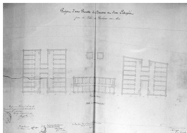
Douane, entrepôt public, plan du sous-sol, éch. 0,01 p.m. B.M. Boulogne-sur-Mer, ms 535 P. pl. 5. Repro. Philippe Dapvril IVR31_19946200055X
