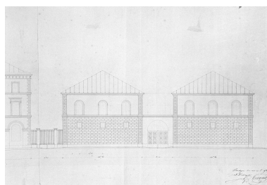
Douane, entrepôt public, façade partielle, partie sud sur quai, plan, éch. 0,01 p.m. B.M. Boulogne-sur-Mer, ms 535 P. pl. 15 partielle. Repro. Philippe Dapvril IVR31_19946200069X
