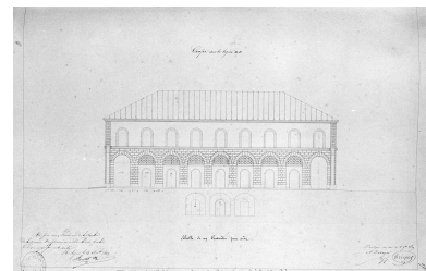
Douane, entrepôt public, coupe E-F, éch. 0,01 p.m. B.M. Boulogne-sur-Mer, ms 535 P. pl. 17. Repro. Philippe Dapvril IVR31_19946200060X
