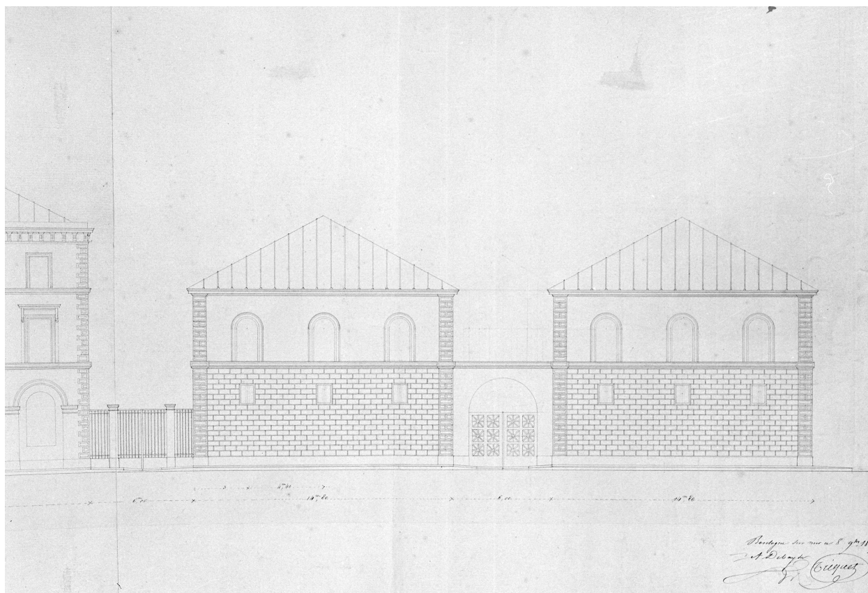
Douane, entrepôt public, façade partielle, partie sud sur quai, plan, éch. 0,01 p.m. B.M. Boulogne-sur-Mer, ms 535 P. pl. 15 partielle.
