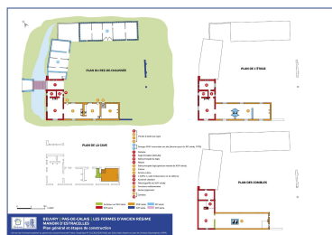
Plan général et chronologie des constructions. Dess. Eddy Stein IVR32_20236200051NUD
