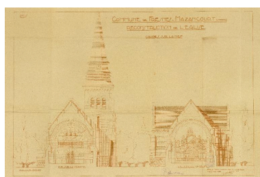
Coupes sur la nef, R. Duthoit (architecte), mai 1928 (AD Somme ; 99 O 1846). Phot. Thierry Lefébure IVR22_20068000513XAB
