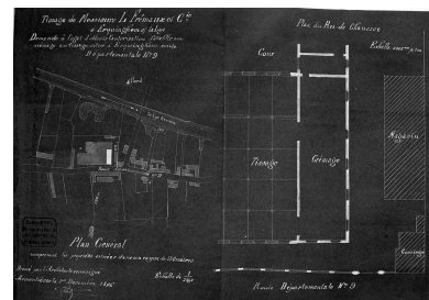
Tissage de messieurs L. Frémaux et Cie. demande d'adjonction d'un crémage au tissage. Plan du rez-de-chaussée, 1896 (AD Nord, M4172458). Repro. Olivier Marlard IVR31_19885901912X
