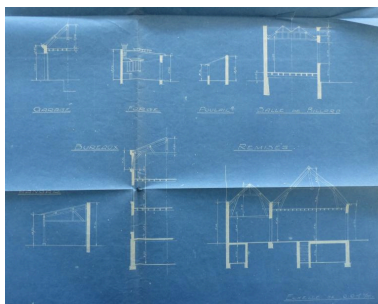
Propriété de M. Outrequin à Villers-Bretonneux. Coupes sur la salle de billard, bureaux, remises et dépendances (AD Somme ; 10R 1272). Phot. Isabelle Barbedor IVR32_20208005291NUCA
