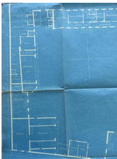
Propriété de M. Outrequin à Villers-Bretonneux. Plan des dépendances, à l'est de la cour (AD Somme ; 10R 1272). Phot. Isabelle Barbedor IVR32_20208005288NUCA
