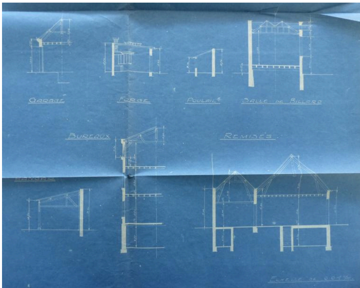
Propriété de M. Outrequin à Villers-Bretonneux. Coupes sur la salle de billard, bureaux, remises et dépendances (AD Somme ; 10R 1272).
