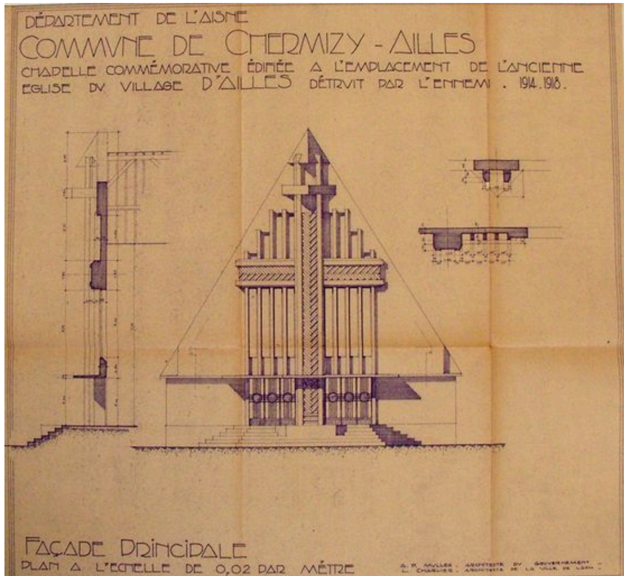
Coupe de la façade principale du projet de la chapelle d'Ailles, par Muller et Charlier (AD Aisne : 15 R 1968).
