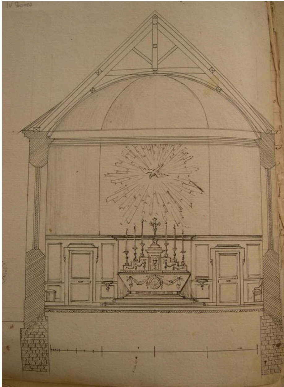
Coupe transversale et vue du chœur, dessin non signé et non daté (AD Somme ; 99 O 847).
