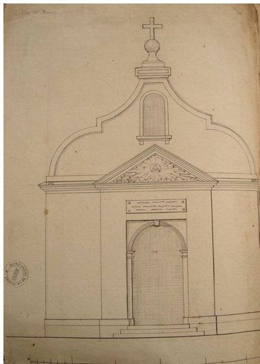
Élévation antérieure, dessin non signé et non daté (AD Somme ; 99 O 847). Phot. Isabelle Barbedor IVR22_20058010400NUCA
