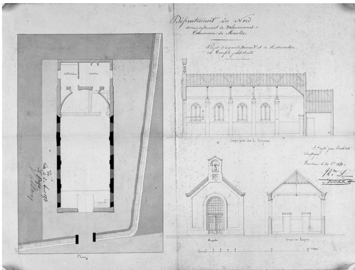
Projet d'agrandissement et de restauration (plan, élévation antérieure, coupes), Lepers architecte, 1854 (AD Nord : 7 V/21).
