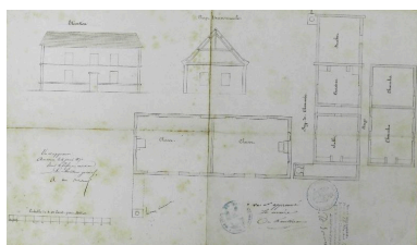
Projet de construction de l'école primaire, 1870 (AD Somme ; 99 O 3366) Phot. Romain Grimaud (reproduction) IVR22_20138016205NUCA
