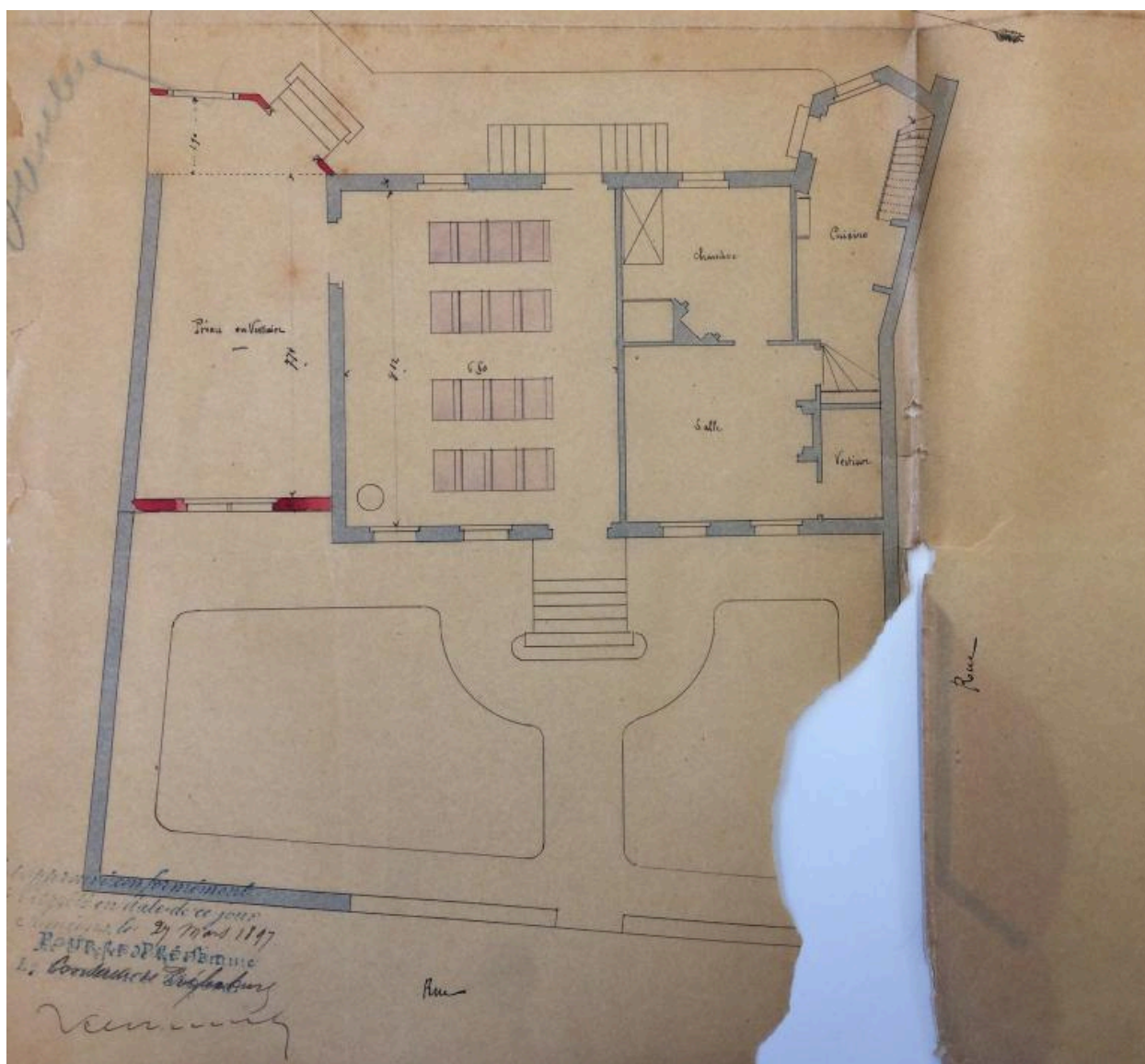
Athies (Somme). Aménagement d'une école enfantine. Plan de la maison d'école, par Darcourt architecte, 1893 (AD Somme ; 99O 427).
