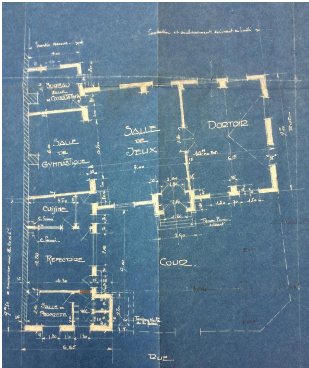
Athies (Somme). Reconstruction de l'école maternelle. Plan du rez-de-chaussée, par E. Chaine architecte, 1929 (AD Somme ; 99O 427).
