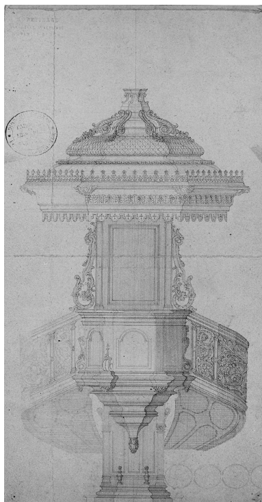
Élévation sur vaisseau central (AD Pas-de-Calais, 9 J 2 OP 100). Repro. Olivier Marlard IVR31_19886200529X
