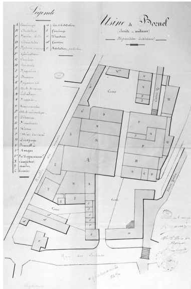
Plan de l'usine de la SFAM, avec détail des bâtiments, 1926 (AD Oise ; Mp 2426). Phot. Thierry Lefébure IVR22_19986000058X
