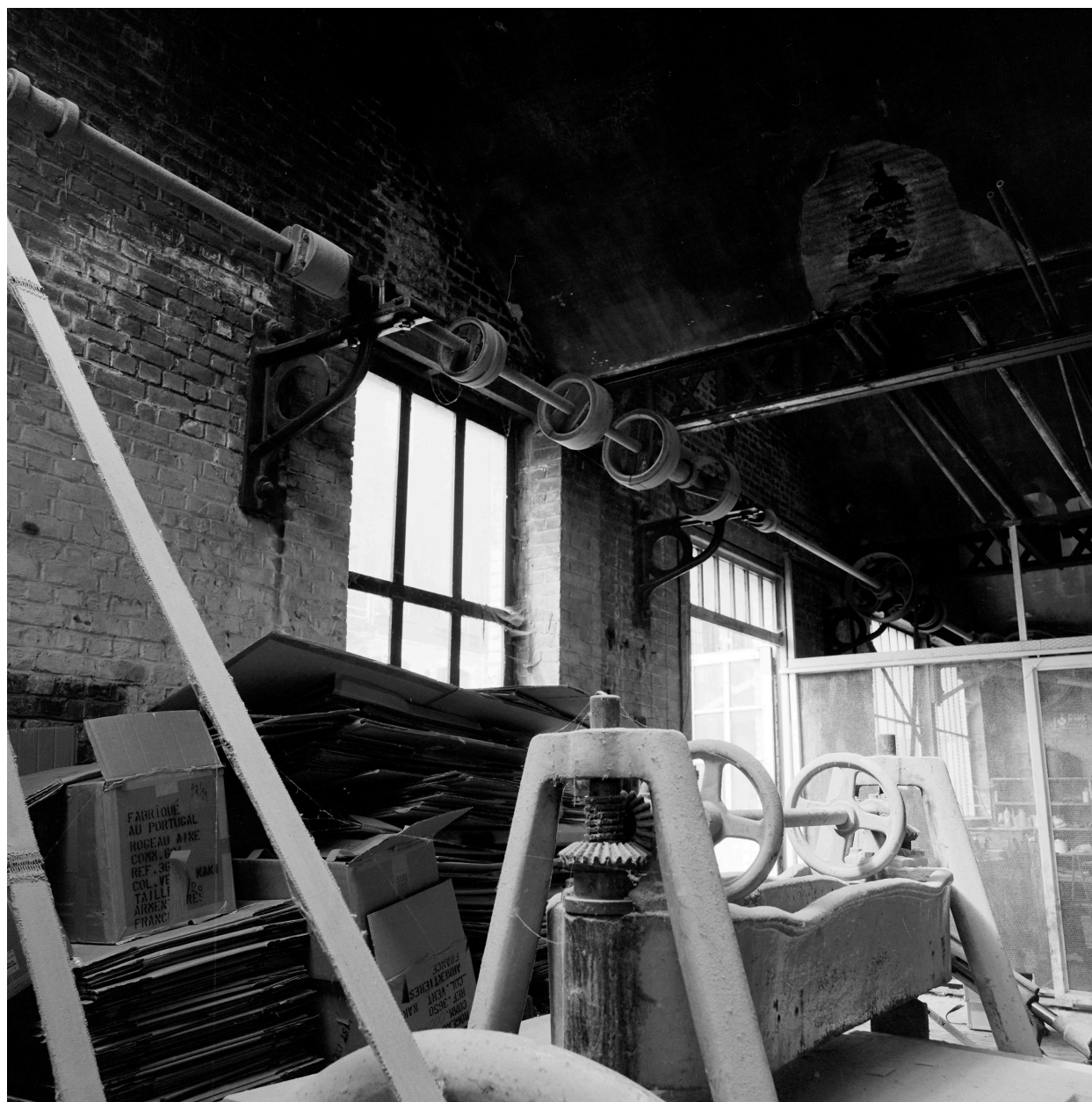
Atelier de fabrication. Presse à découper le cuir, axe de transmission.
