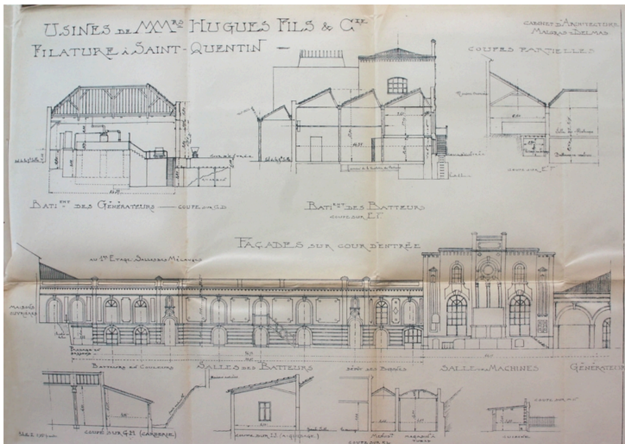
Façades et coupes de la filature en 1914, par Malgras-Delmas (AD Aisne).
