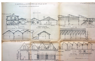
Façades et coupes de la filature en 1914, par Malgras-Delmas (AD Aisne). Phot. Pillet Frédéric IVR22_20060205397NUCAB
