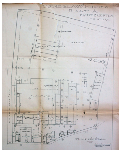
Plan général de l'usine en 1914, par Malgras-Delmas (AD Aisne). Phot. Pillet Frédéric IVR22_20060205394NUCAB
