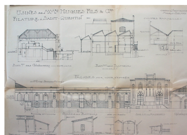
Façades et coupes de la filature en 1914, par Malgras-Delmas (AD Aisne). Phot. Pillet Frédéric IVR22_20060205396NUCAB
